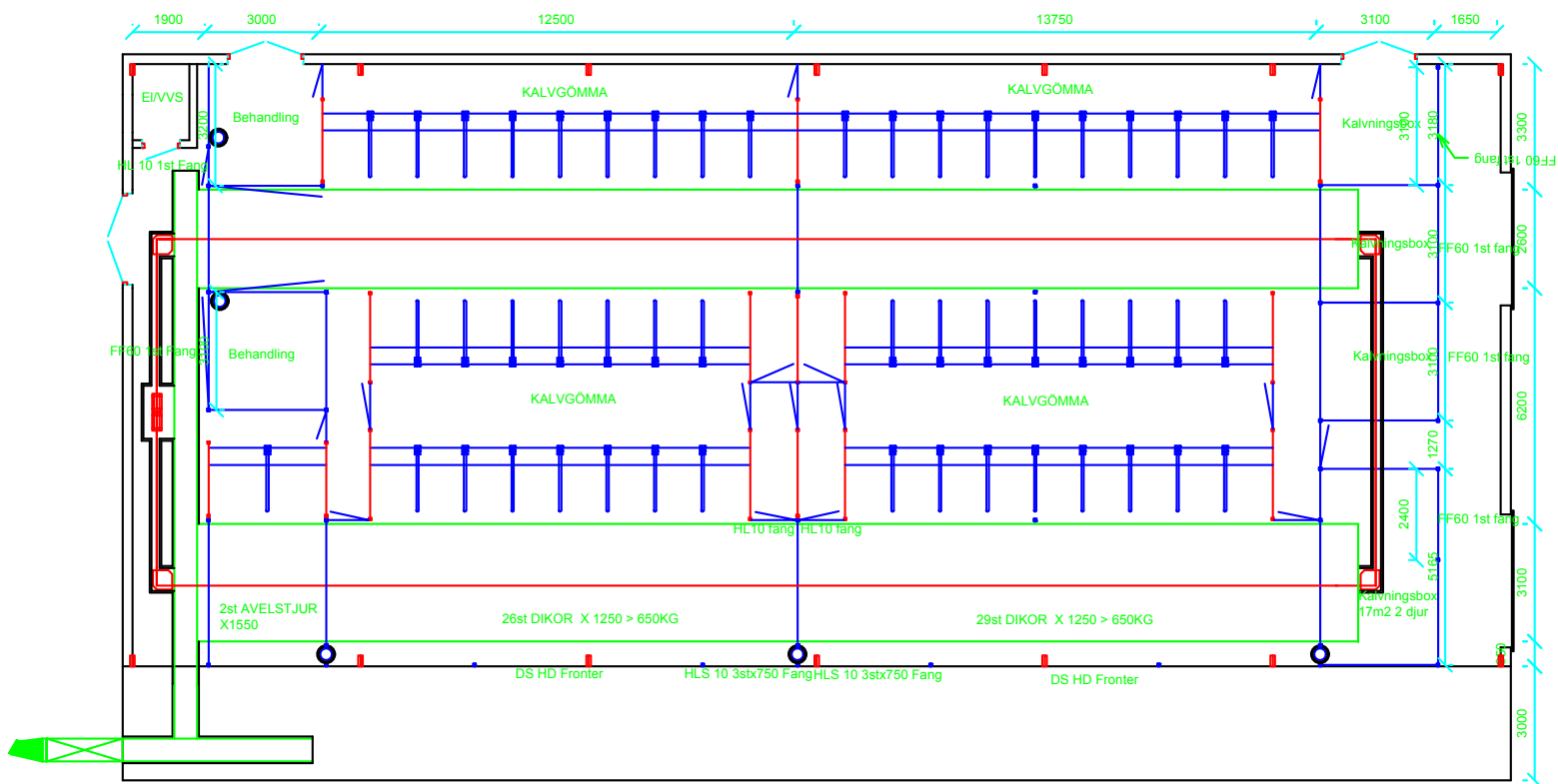
Ritningen av stallet på Kråkenäs Säteri.
