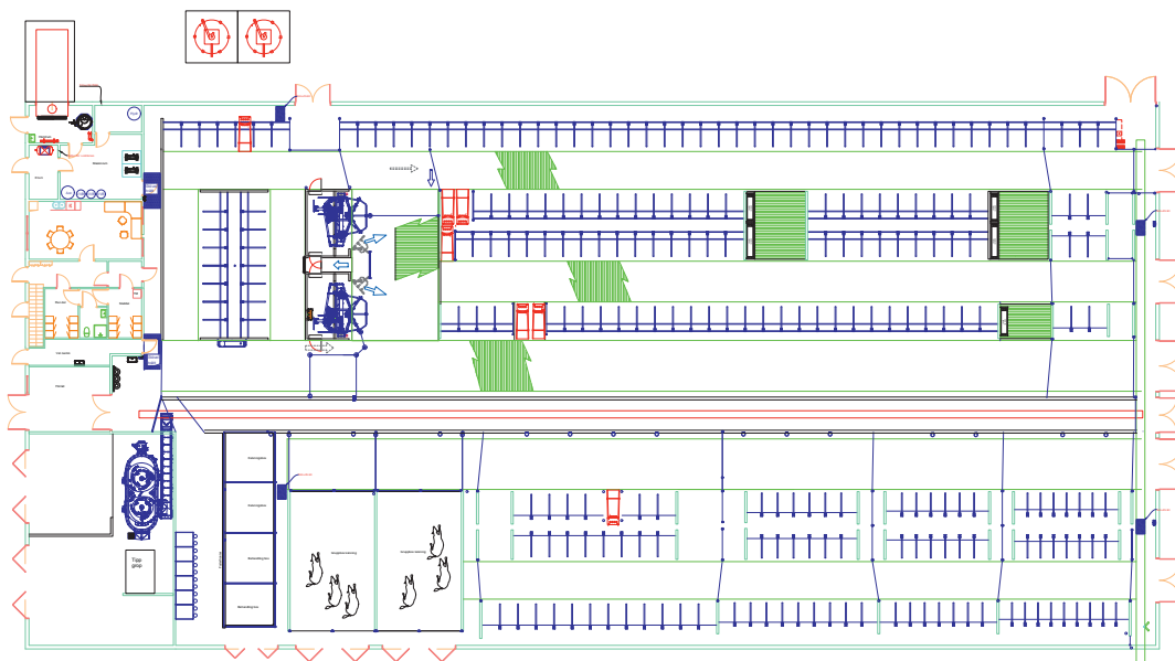
Exempel 2: Stall med två DeLaval VMS™ V300 och Optimat™ Standard med bandfoderfordelare.
