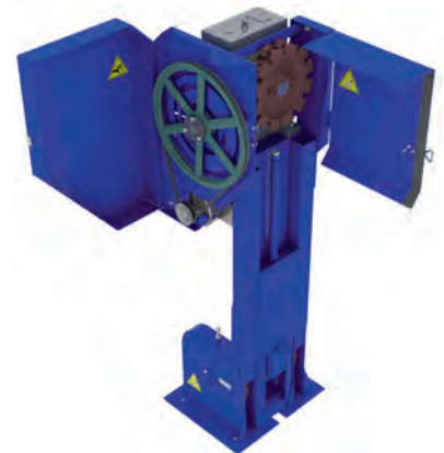
Drivenhet till AKD140 med öppna luckor
